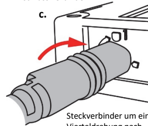
Steckverbinder unter Beachtung des Diagramms auf dem Logger-Gehäuse (s. oben) mit dem Analogsensor-Anschluss verbinden.
